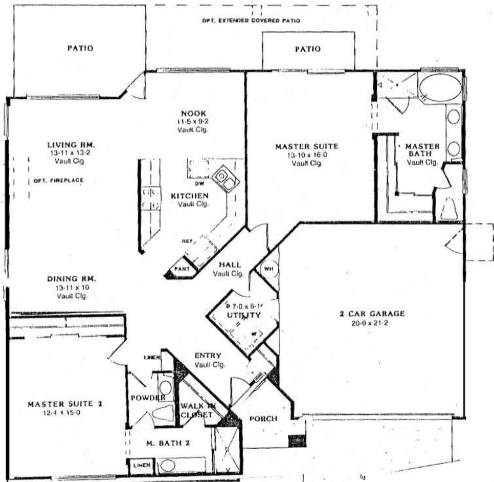
723-3 ESTRELLA (3-BEDROOM)
